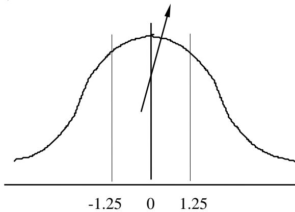
Gambar 8. Peluang ( -1.25 < z < 1.25 )
