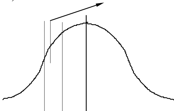
Gambar 8. Peluang ( -1.25 < z < 1.25 )
