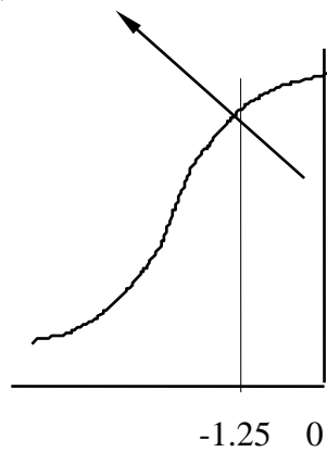
Gambar 5. Peluang ( -1.25 < z < 0 )
