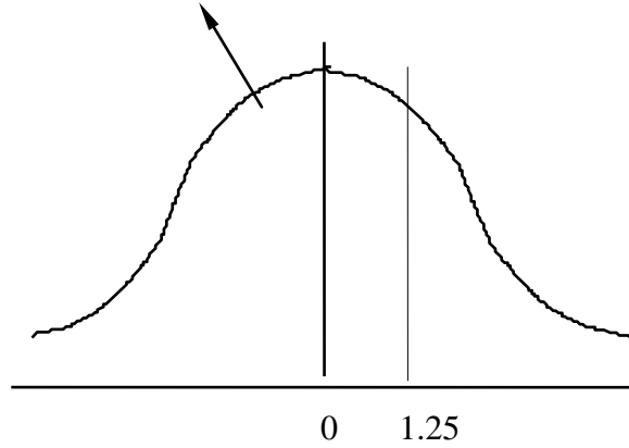
Gambar 4. Peluang ( z < 1.25 )
