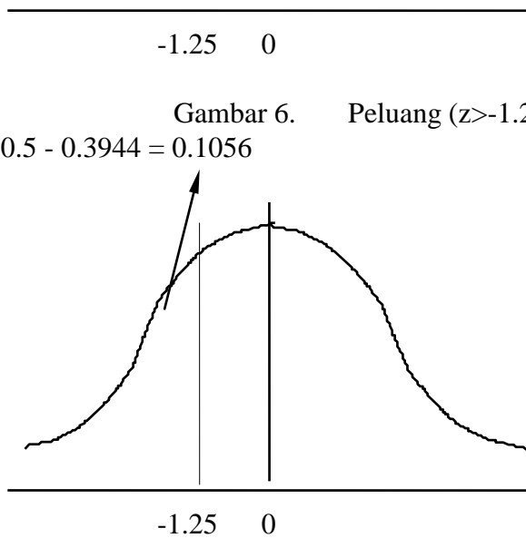
Gambar 7. Peluang ( z < -1.25 )
